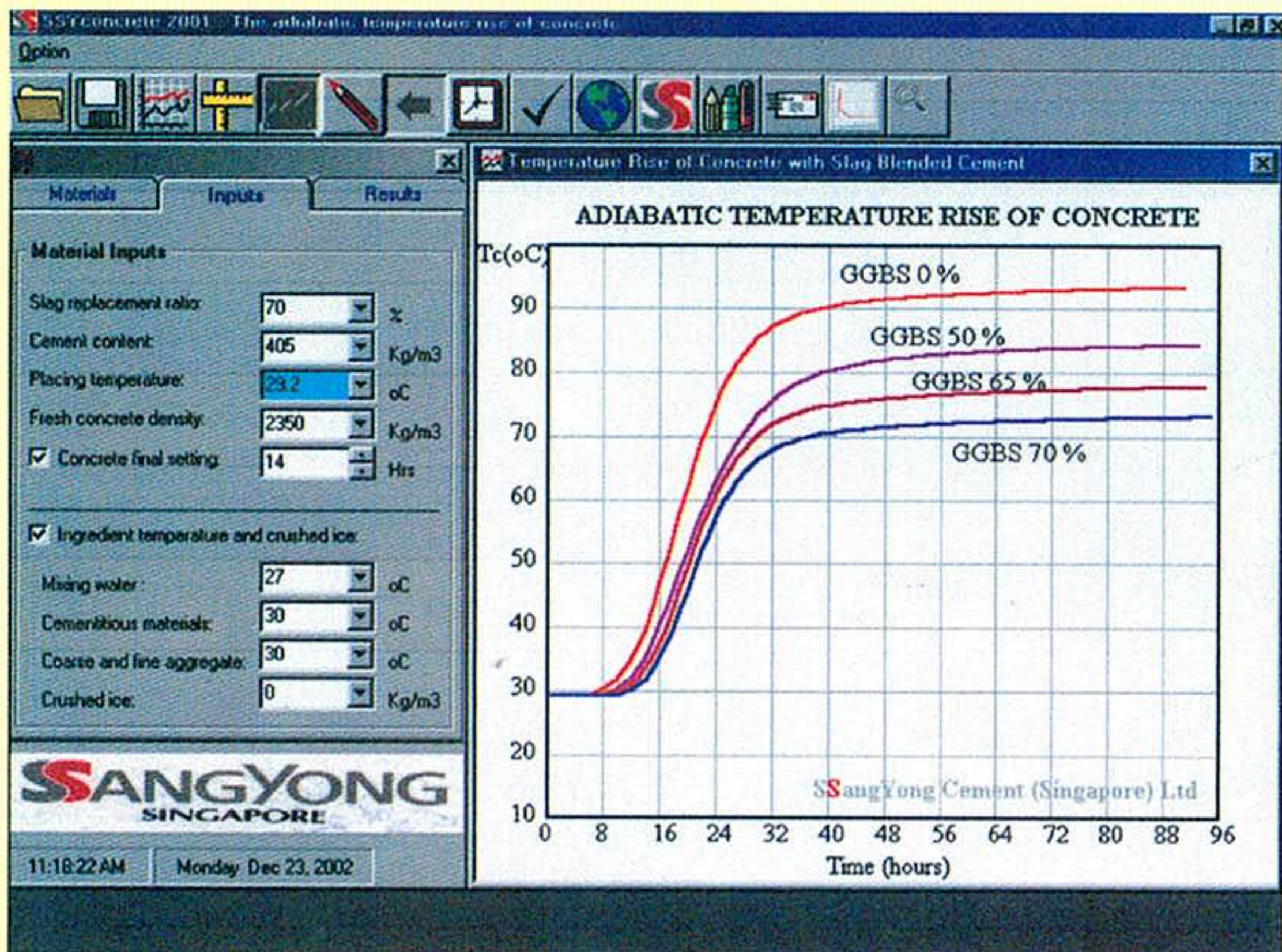
矿粉(GGBS)掺量对绝热条件下混凝土中心温度的影响 (计算机模拟结果)
