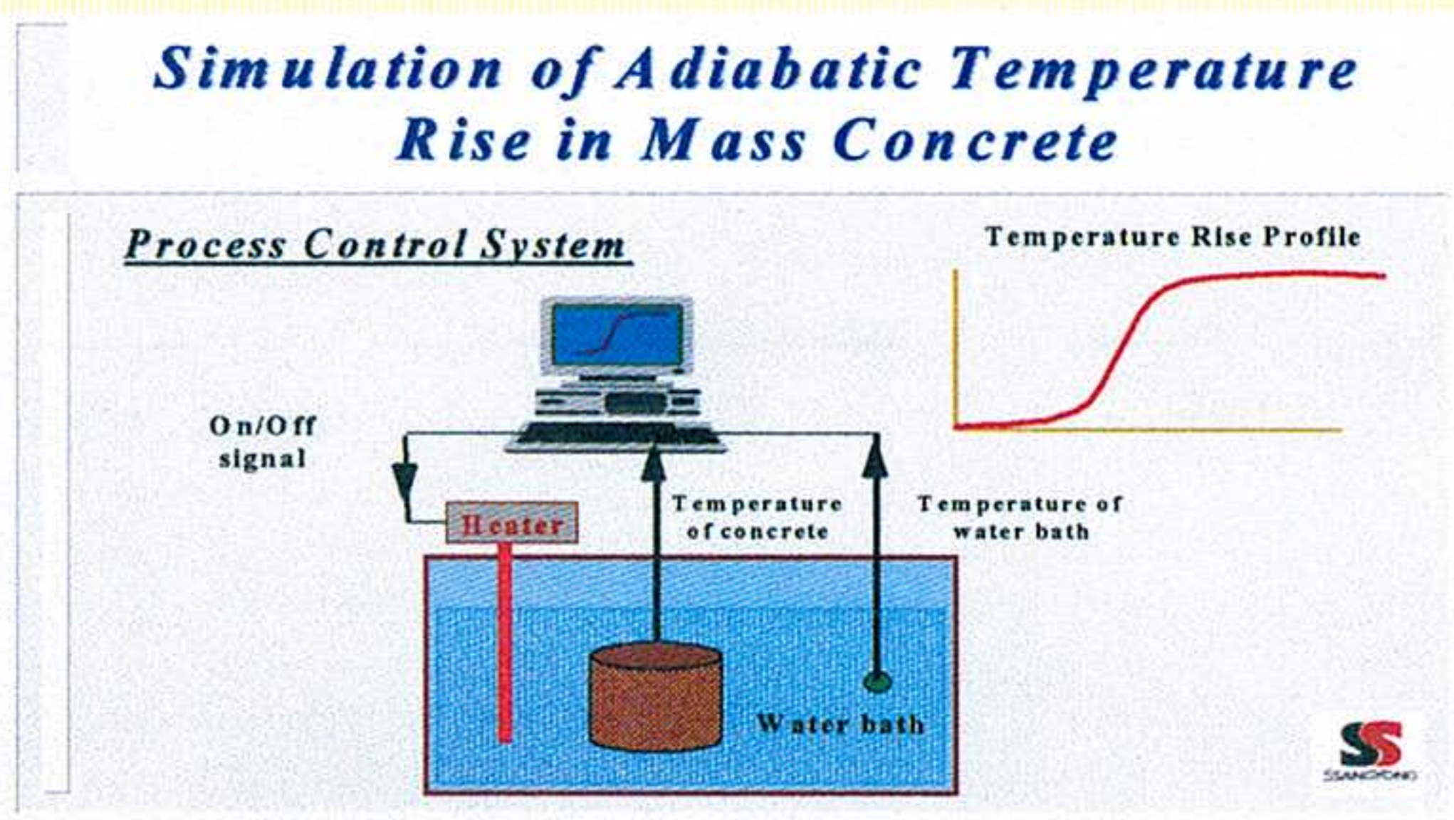
大体积混凝土温升模拟测试系统
