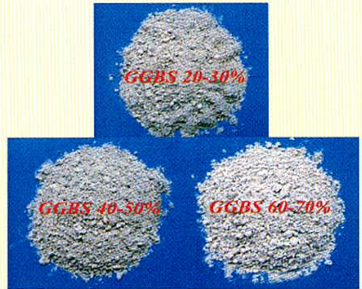
“伟胜”牌普通及大掺量矿渣水泥 (PBFC&HSPBFC)
